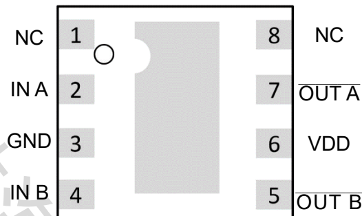
SOP8
