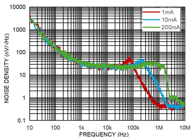
图 14. 噪声谱密度
