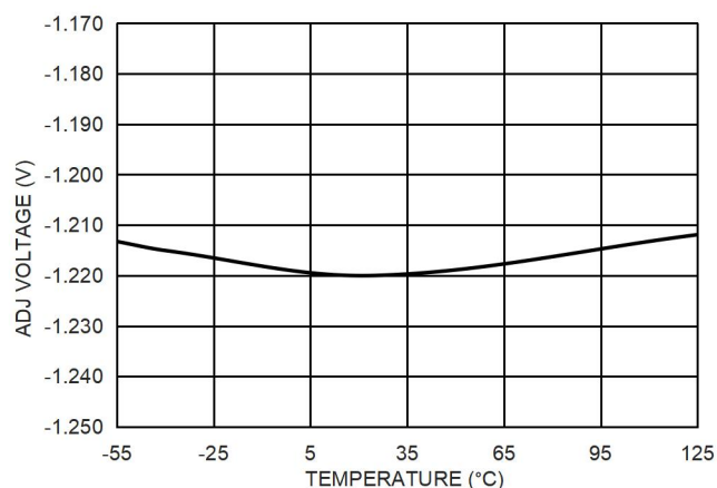
图 8. ADJ 引脚电压与结温 ( T_j ) 的关系
