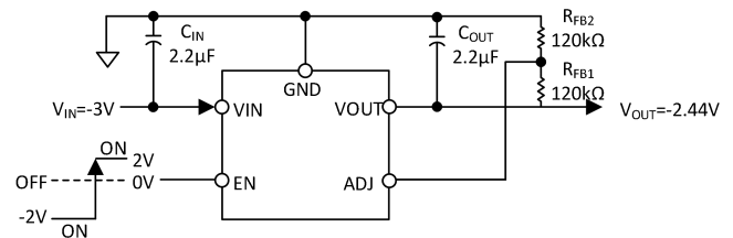
图 1 典型应用
