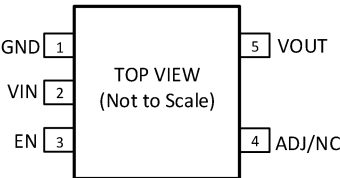
图 4. SOT-23 引脚配置(顶视图)
