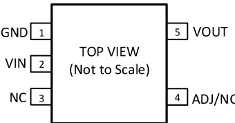
图 5. SOT-23 引脚配置(顶视图)
