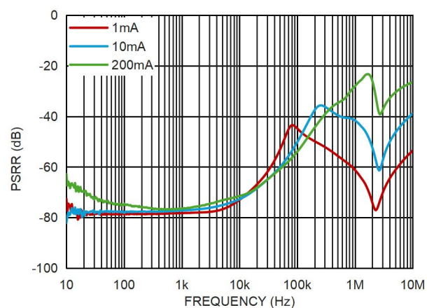
图 16. PSRR 和负载电流的关系
