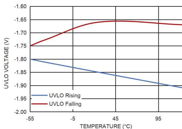
图 17. UVLO 阈值和结温的关系
