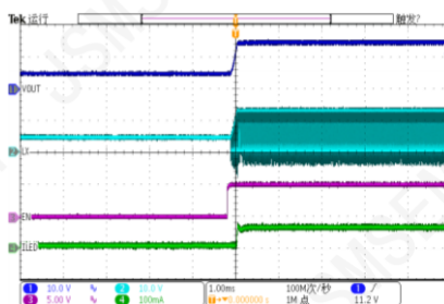
Enable Startup
