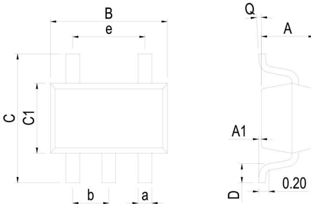
SOT-23-5
