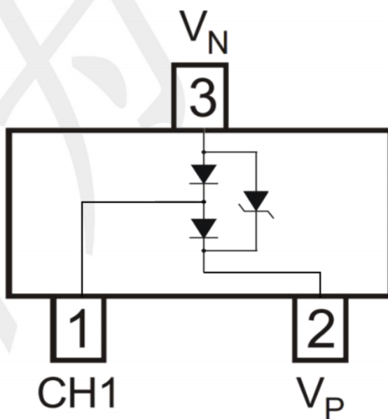
SOT-323
