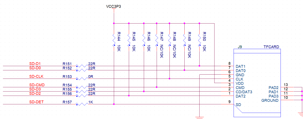
图 19 TF 卡电路
