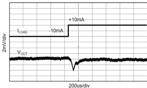
图 8 Load Transient @VIN=5V, CL=10uF, 负载 20mA 阶跃变化上升
