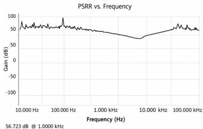
图 11 PSRR 曲线
