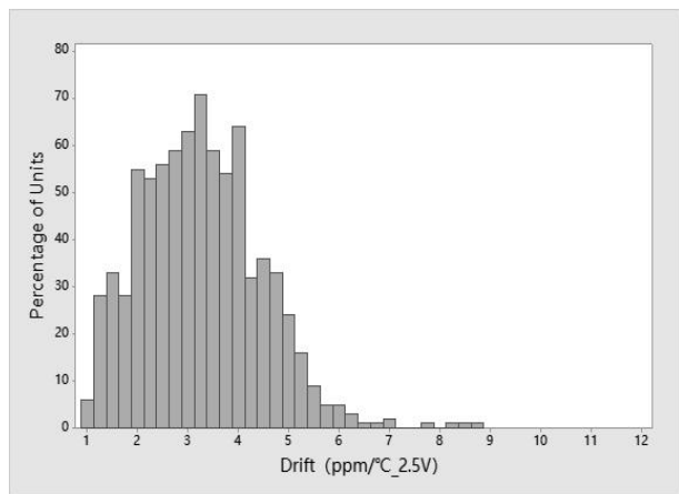
图 13 温漂占比
