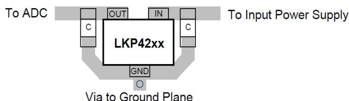
图 23 布局示意图
