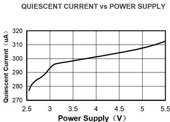
图 15 静态电流与电源电压关系曲线
