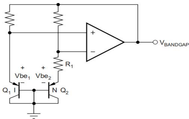
图 14 功能框图
