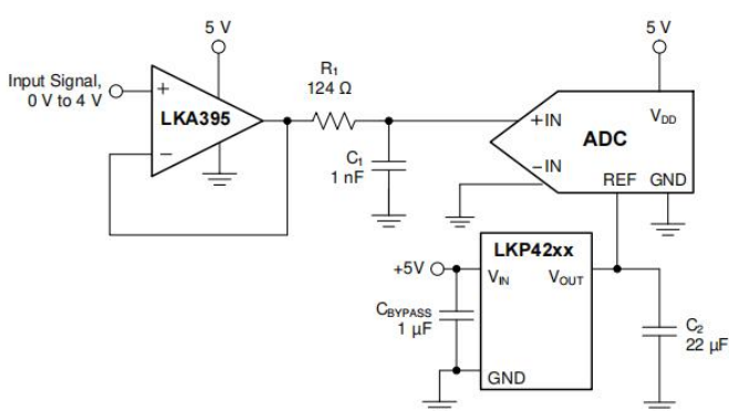
图 1 典型应用图
