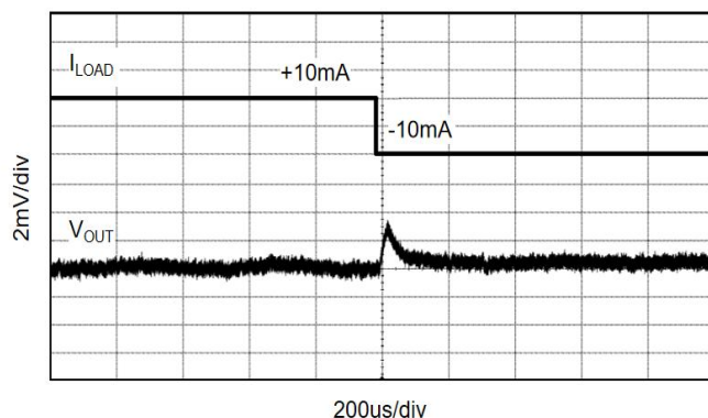
图 9 VIN=5V, CL=10uF, 负载 20mA 阶跃变化下降
