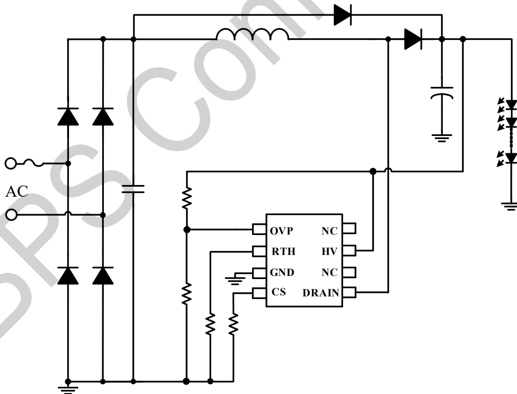
图 1 BP2616B 典型应用电路
