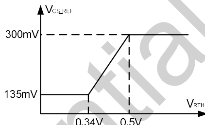
图 6 NTC 降功率曲线
