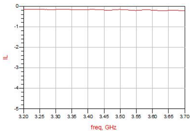
Figure 11. MHC35X02 IL
