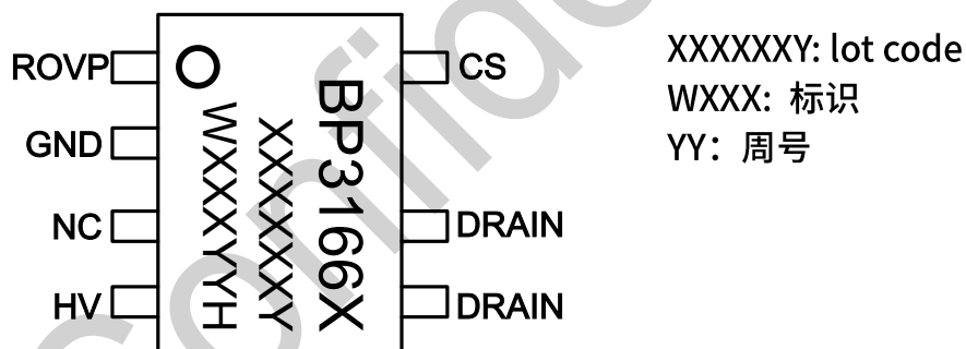
图 2 管脚封装图
