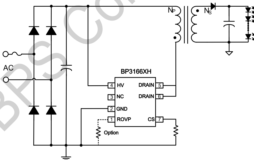
图 1 BP3166XH 典型应用图
