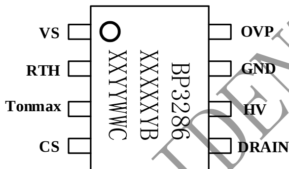
图 2 管脚封装图
