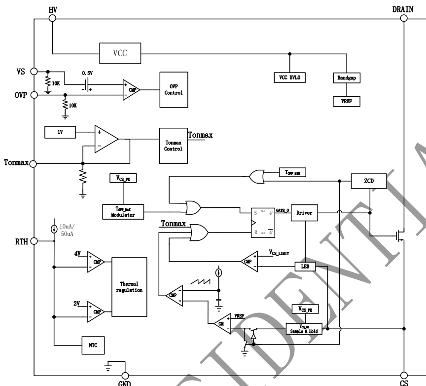
图 3 BP3286CB 内部框图
