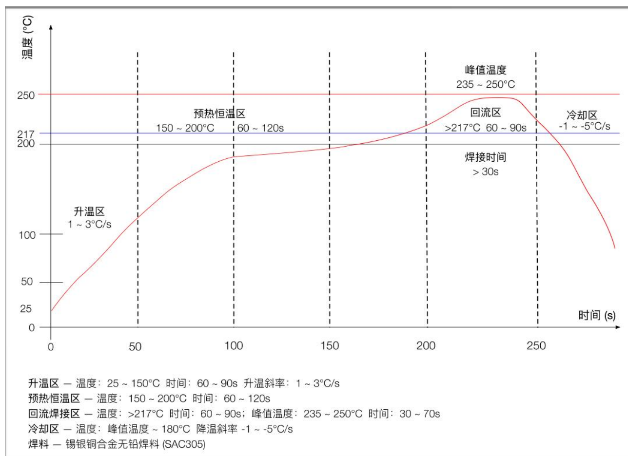
图 12 回流焊曲线
