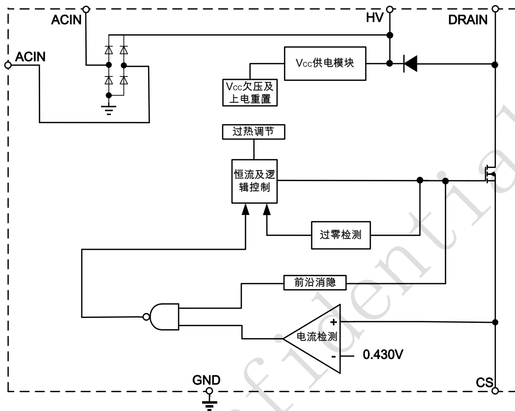
图 3 BP2863MC 内部框图
