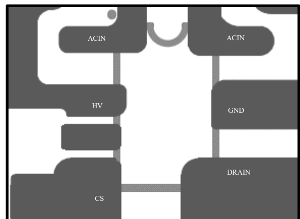
图 4 PCB 铺铜面积优化图
