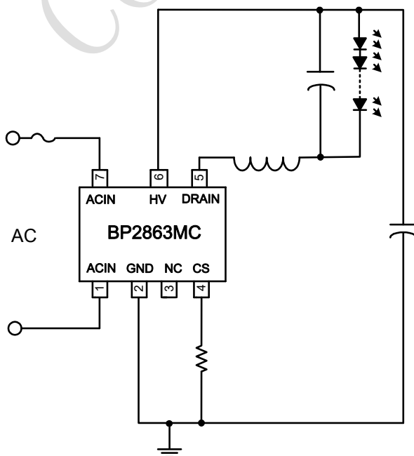
图 1 BP2863MC 典型应用图
