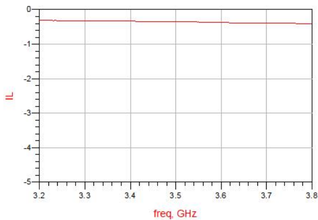
Figure 11. MHC35X03 IL
