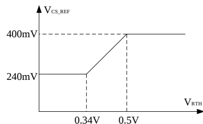
图 7. NTC 降功率曲线
