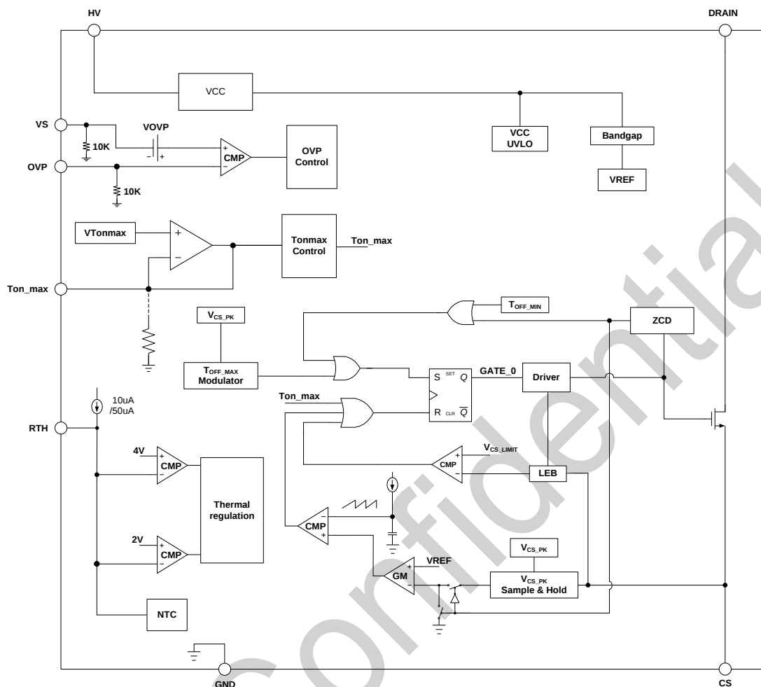
图 3. BP3287HL 内部框图
