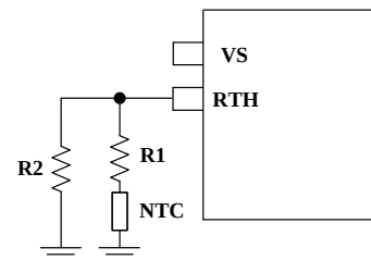
图 6. NTC 参考线路
