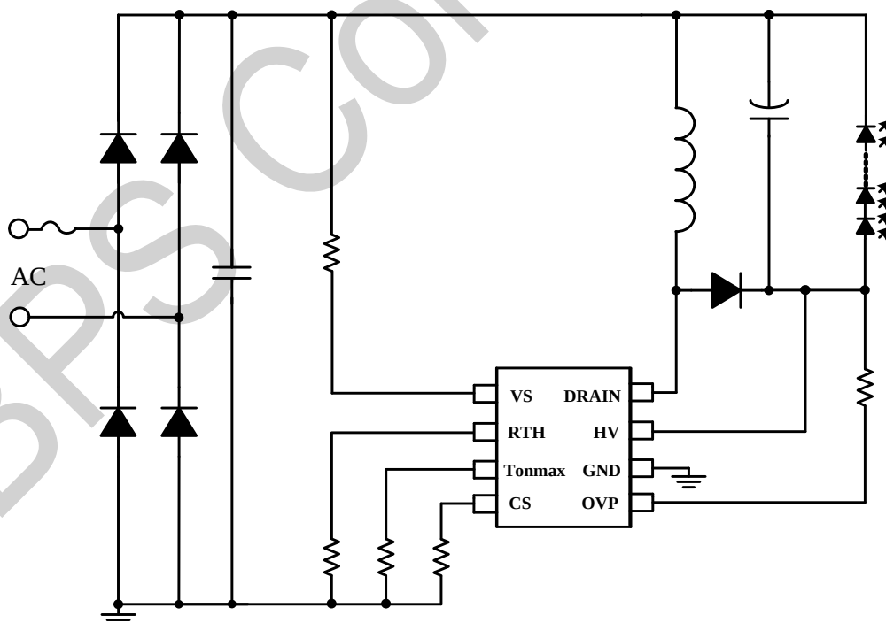
图 1. BP3287HL 典型应用图 (Buck-Boost)
