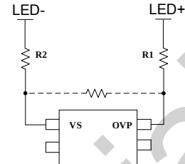
图 5. OVP 线路示意图
