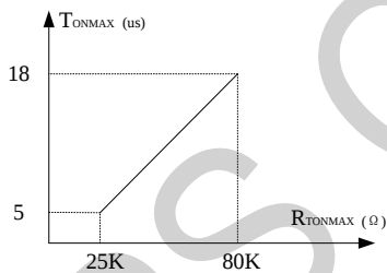
图 4. Tonmax 设置曲线
