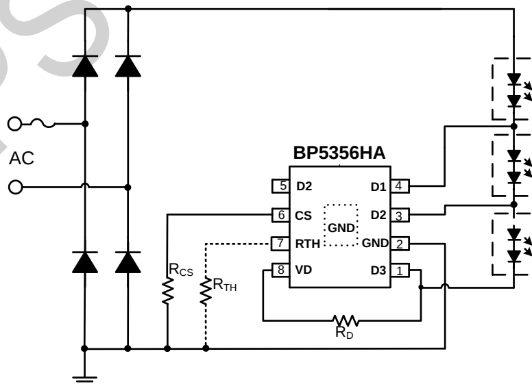
图 1 BP5356HA 典型应用图
