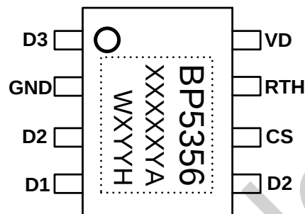
图 2 管脚封装图
