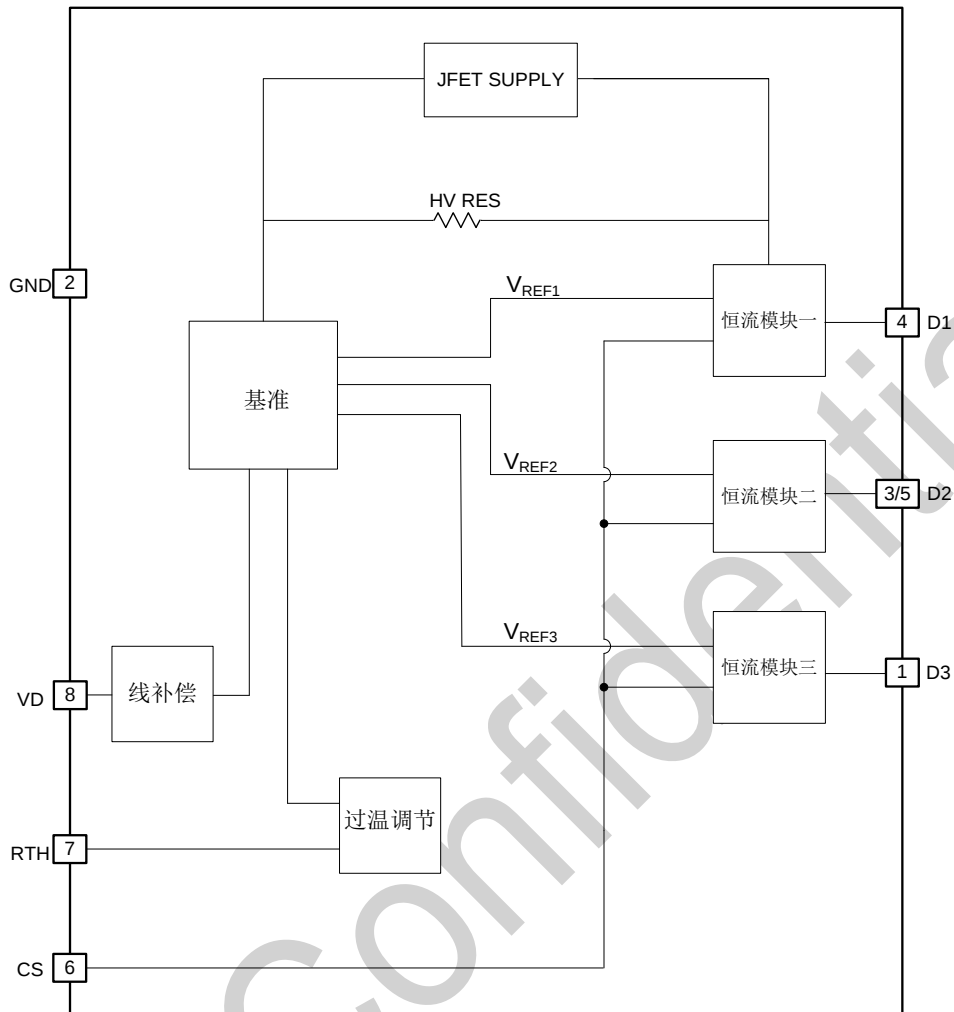
图 3 BP5356HA 内部框图
