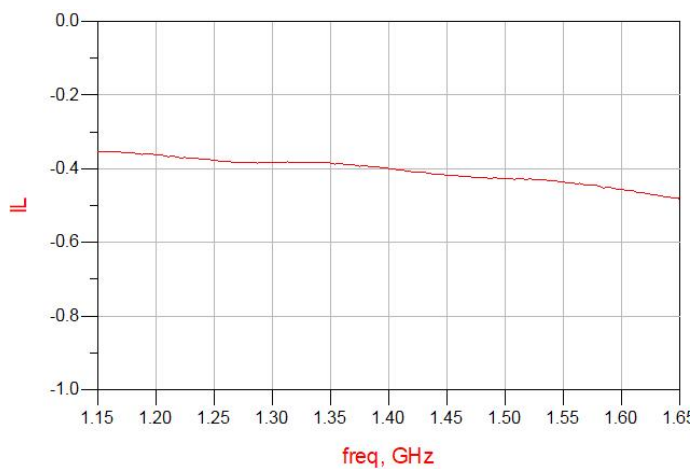
Figure 11. MHC14S03 IL
