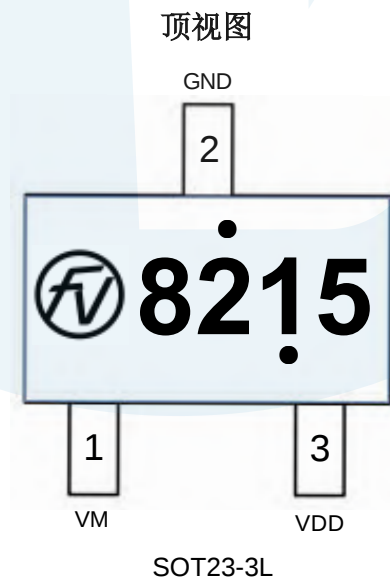
图 1. 引脚定义图
