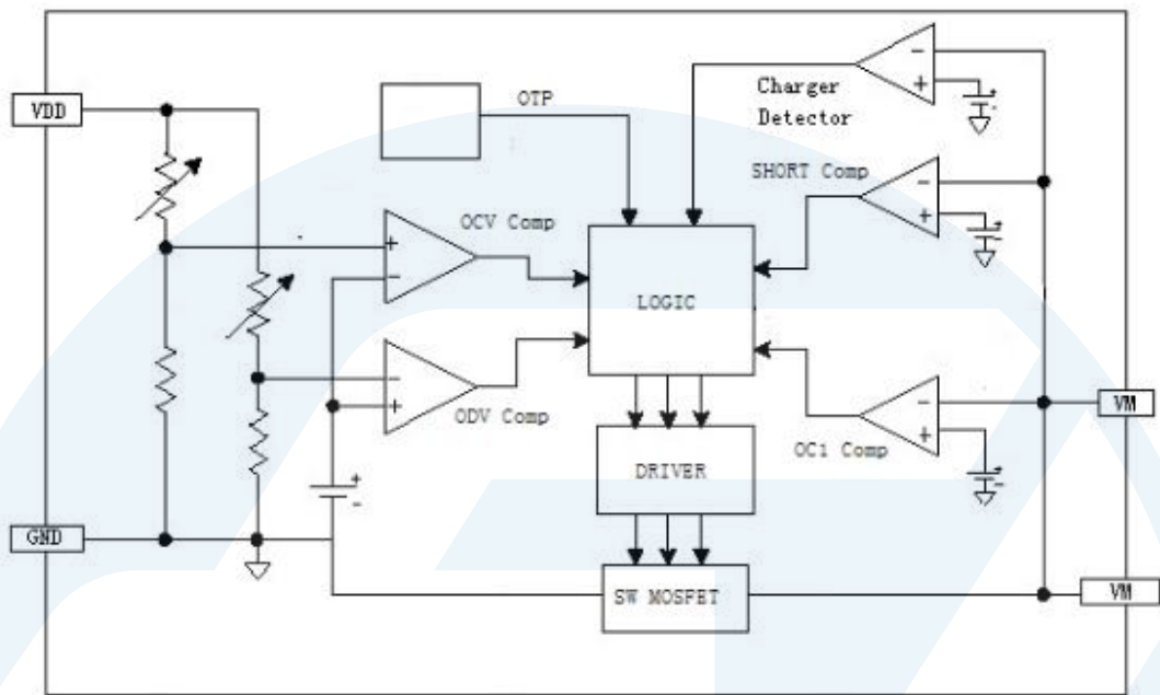
Figure 1. 原理图
