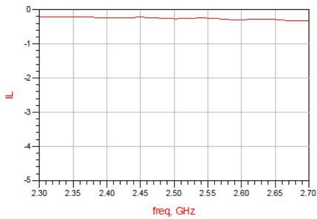
Figure 11. MHC25X02 IL
