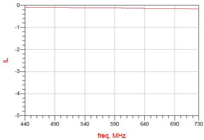
Figure 11. MHC0600L03 IL
