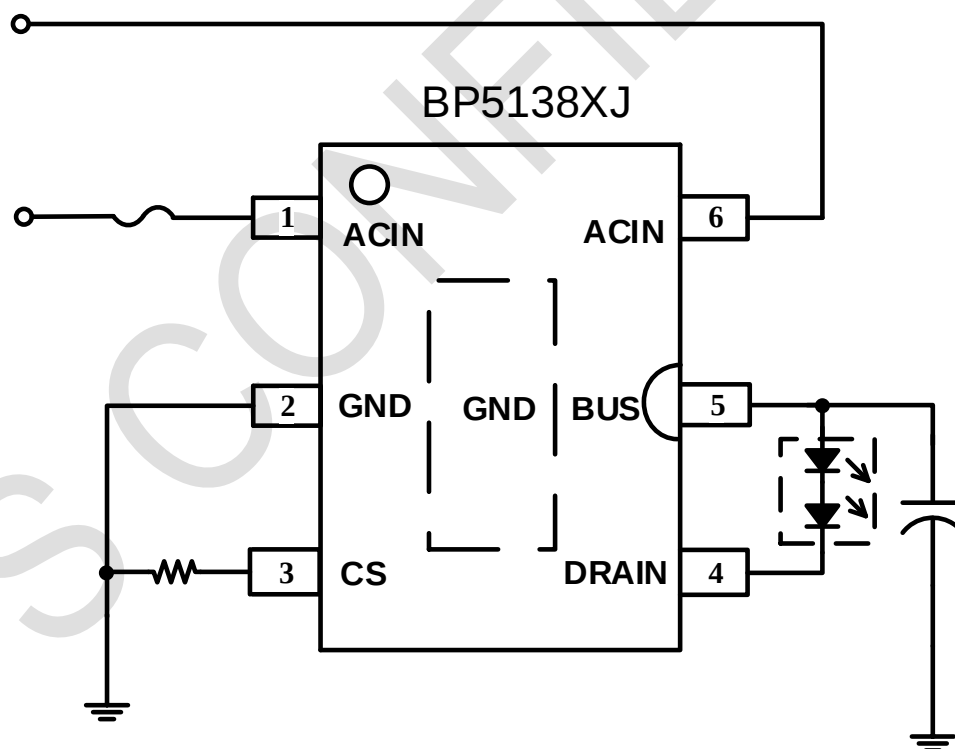
图 1 BP5138XJ 典型应用图
