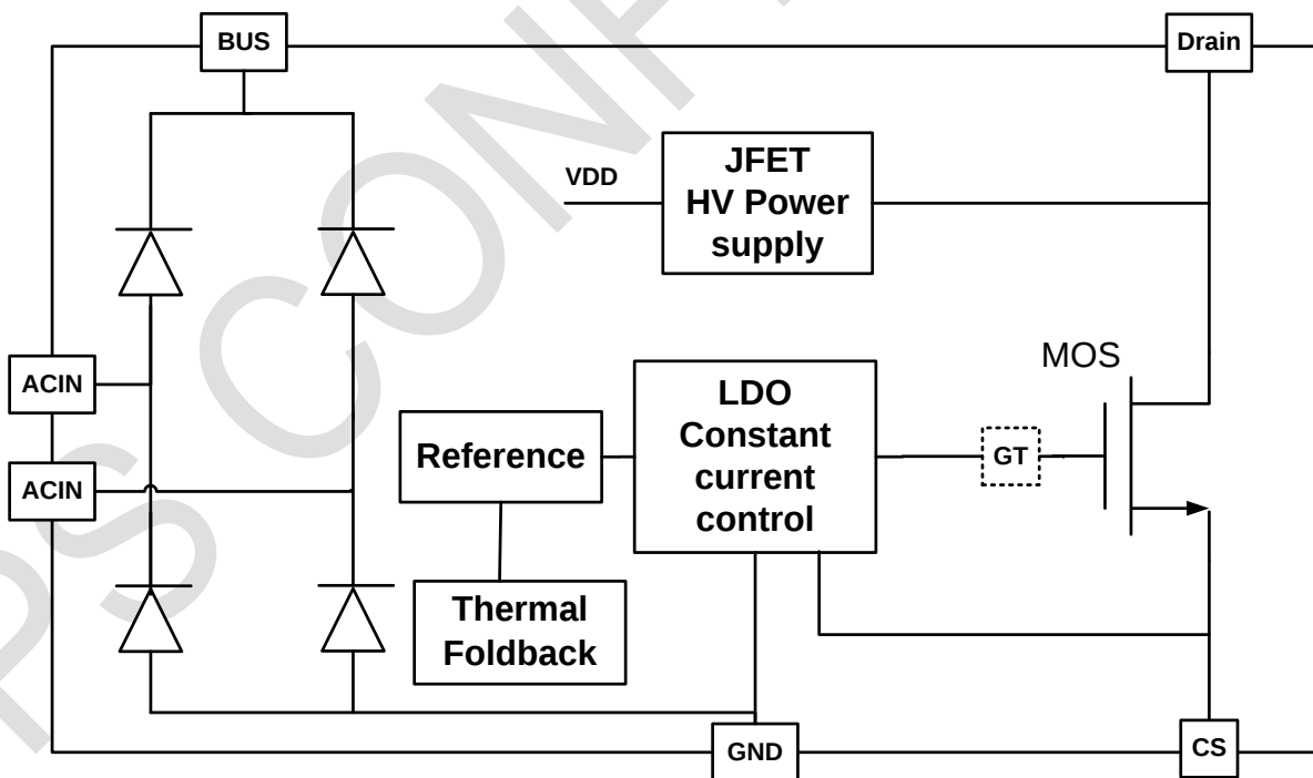
图 3 BP5138XJ 部框图
