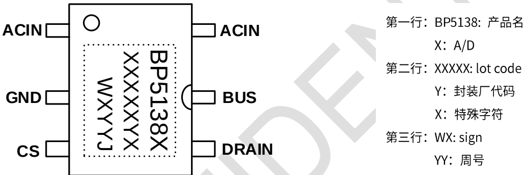
图 2 BP5138XJ 管脚封装图
