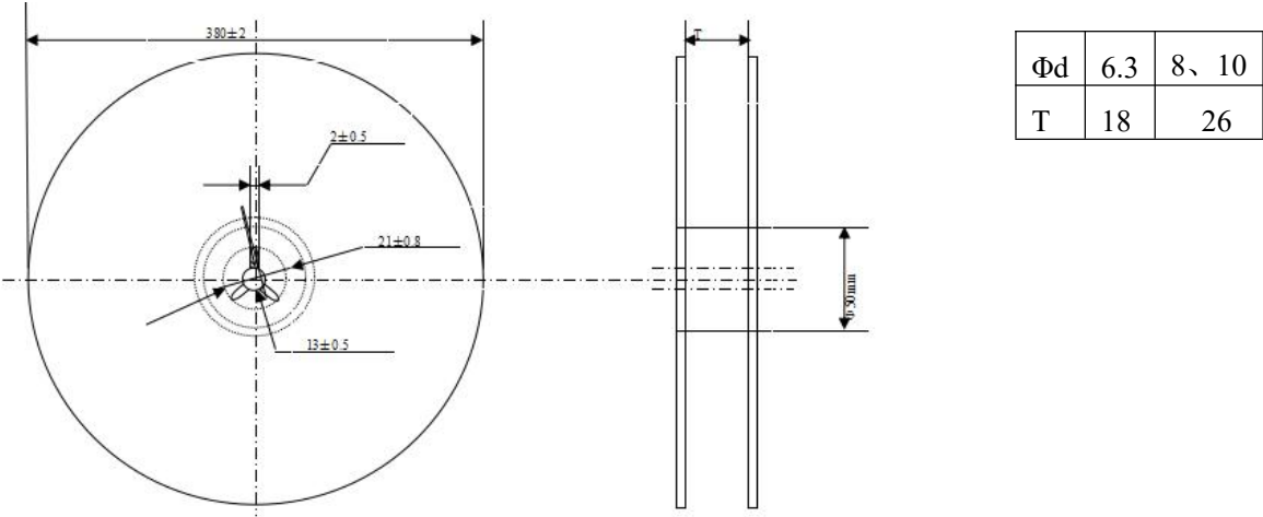
编带包装盘 (mm)
