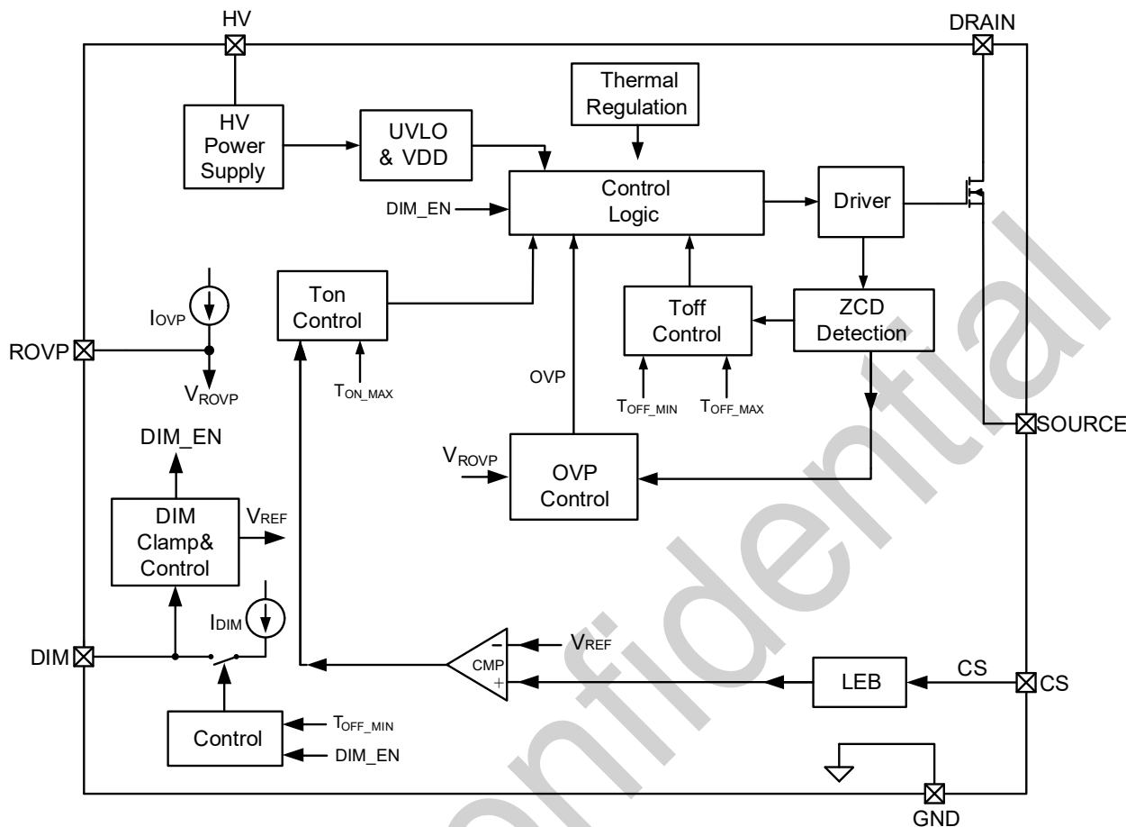
图 3 BP2872GS 内部框图
