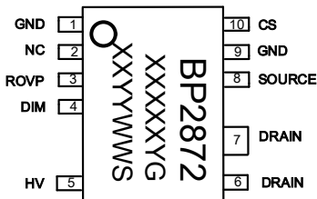
图 2 管脚封装图
