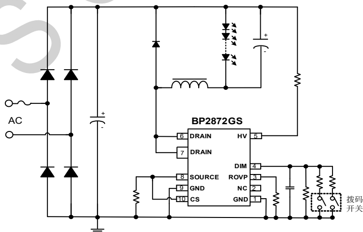
图 1 BP2872GS 典型应用电路
