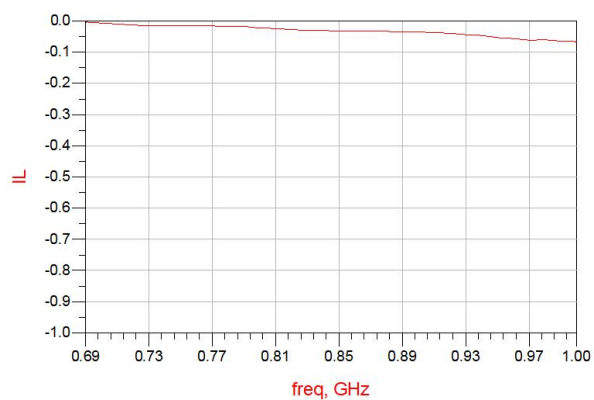
Figure 10. MHC0900L03 IL
