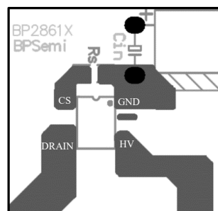
图 4 PCB 铺铜面积优化图
