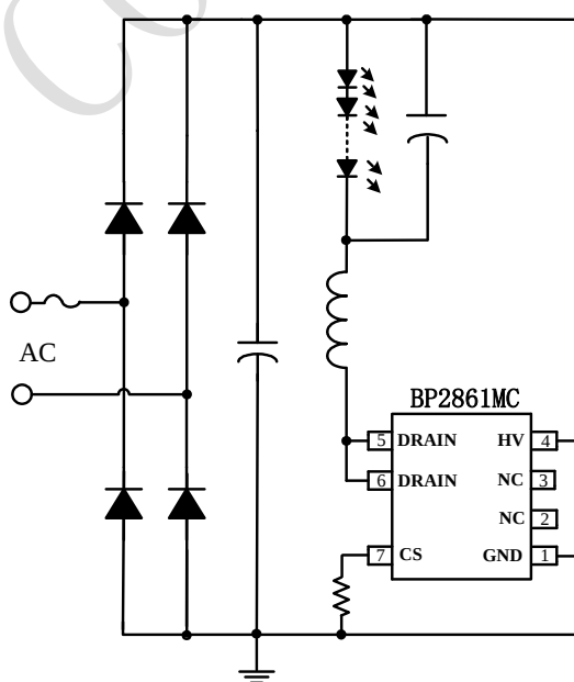
图 1 BP2861MC 典型应用图
