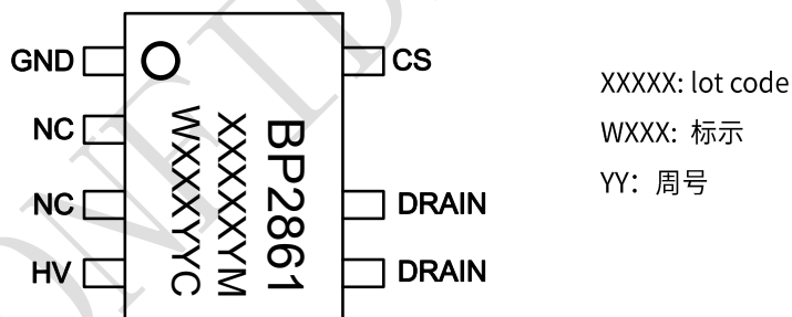
图 2 管脚封装图
