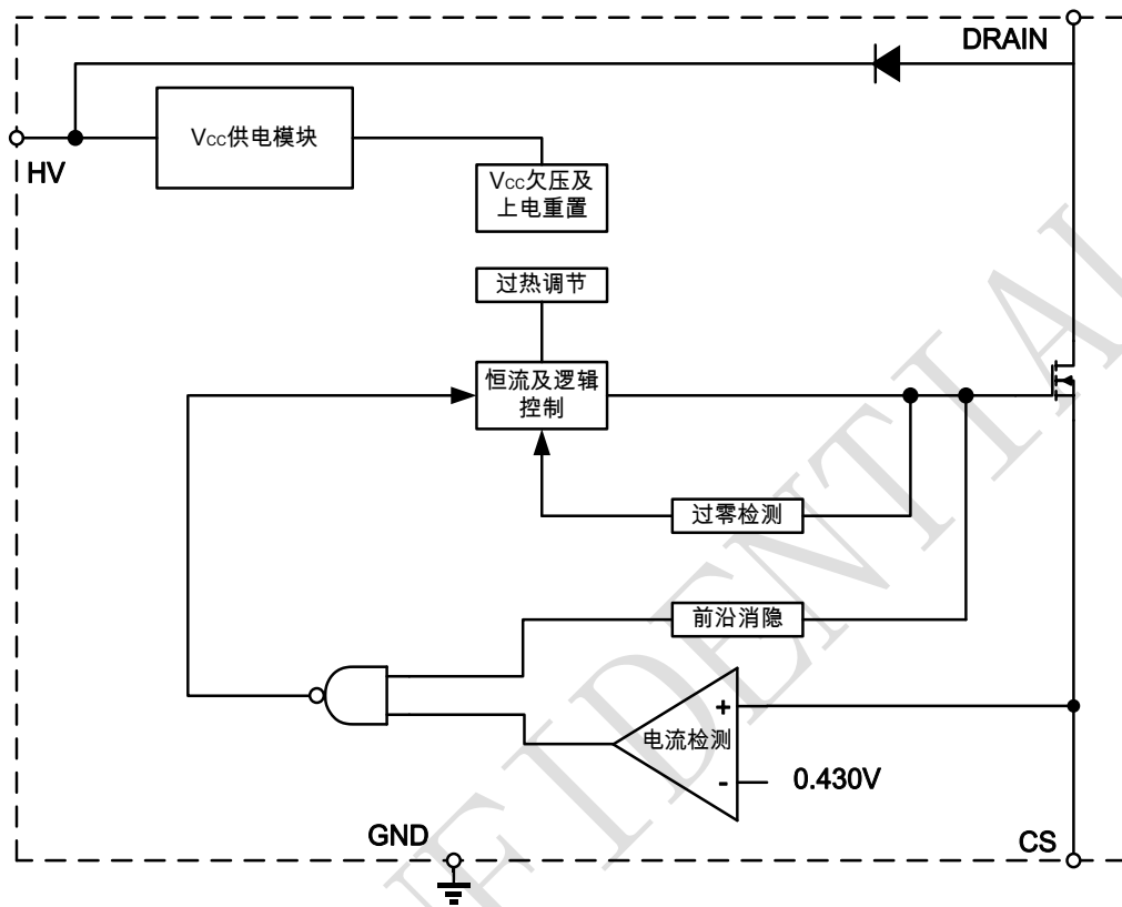
图 3 BP2861MC 内部框图
