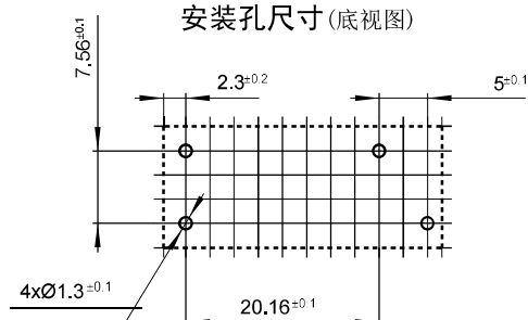
安装孔尺寸(底视图)
