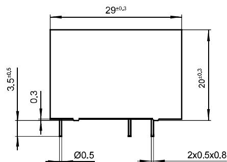
外形图
