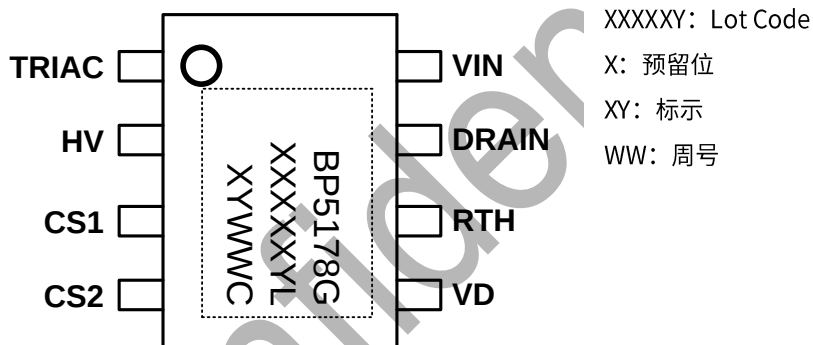
图 2 管脚封装图
