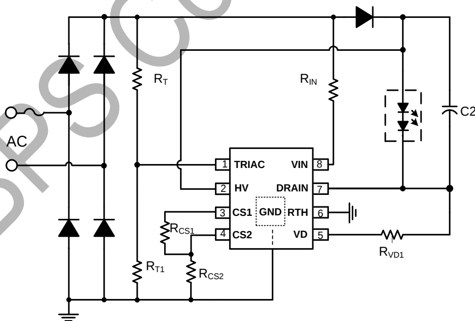
图 1 BP5178GCL 典型应用图
