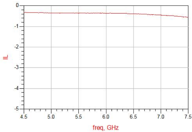
Figure 11. MHC60X03 IL
