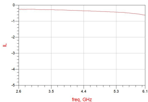
Figure 11. MHC4350L03 IL
