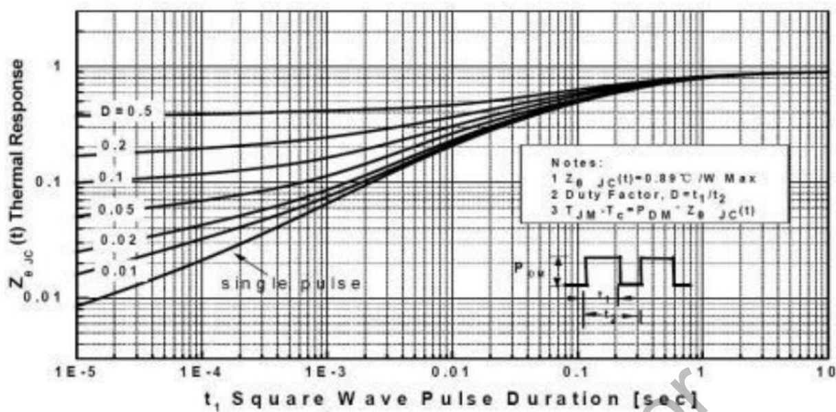
图7. 瞬态热响应曲线(TO-220)
