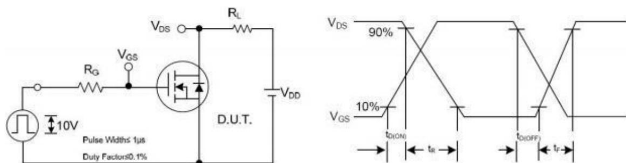
图9. 开关特性测试
