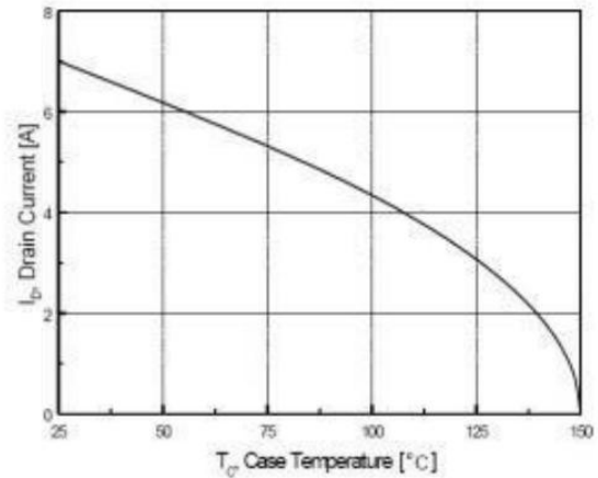
图6. 最大漏极电流随温度变化曲线
