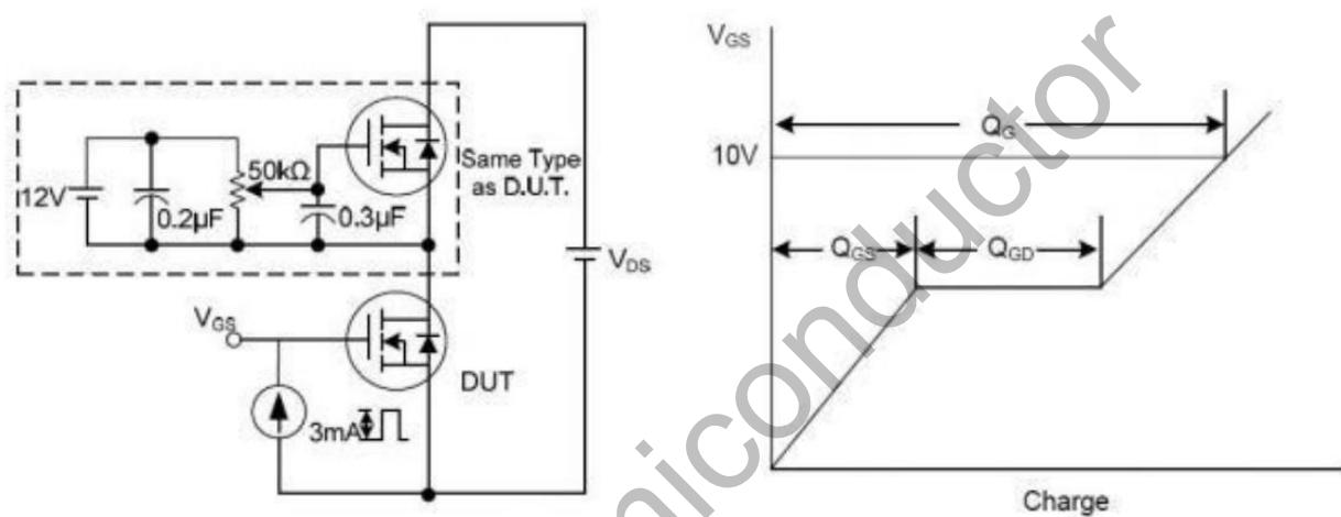
图10. 栅电荷测试
