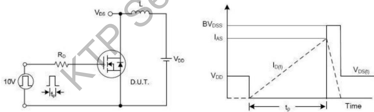
图11. 雪崩能量测试
