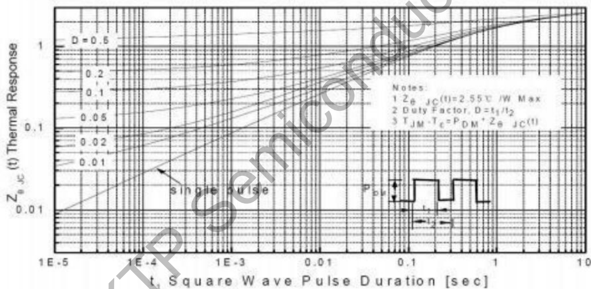
图8. 瞬态热响应曲线(TO-220F)
