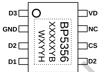
图 2 管脚封装图
