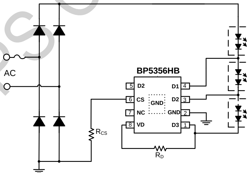
图 1 BP5356HB 典型应用图
