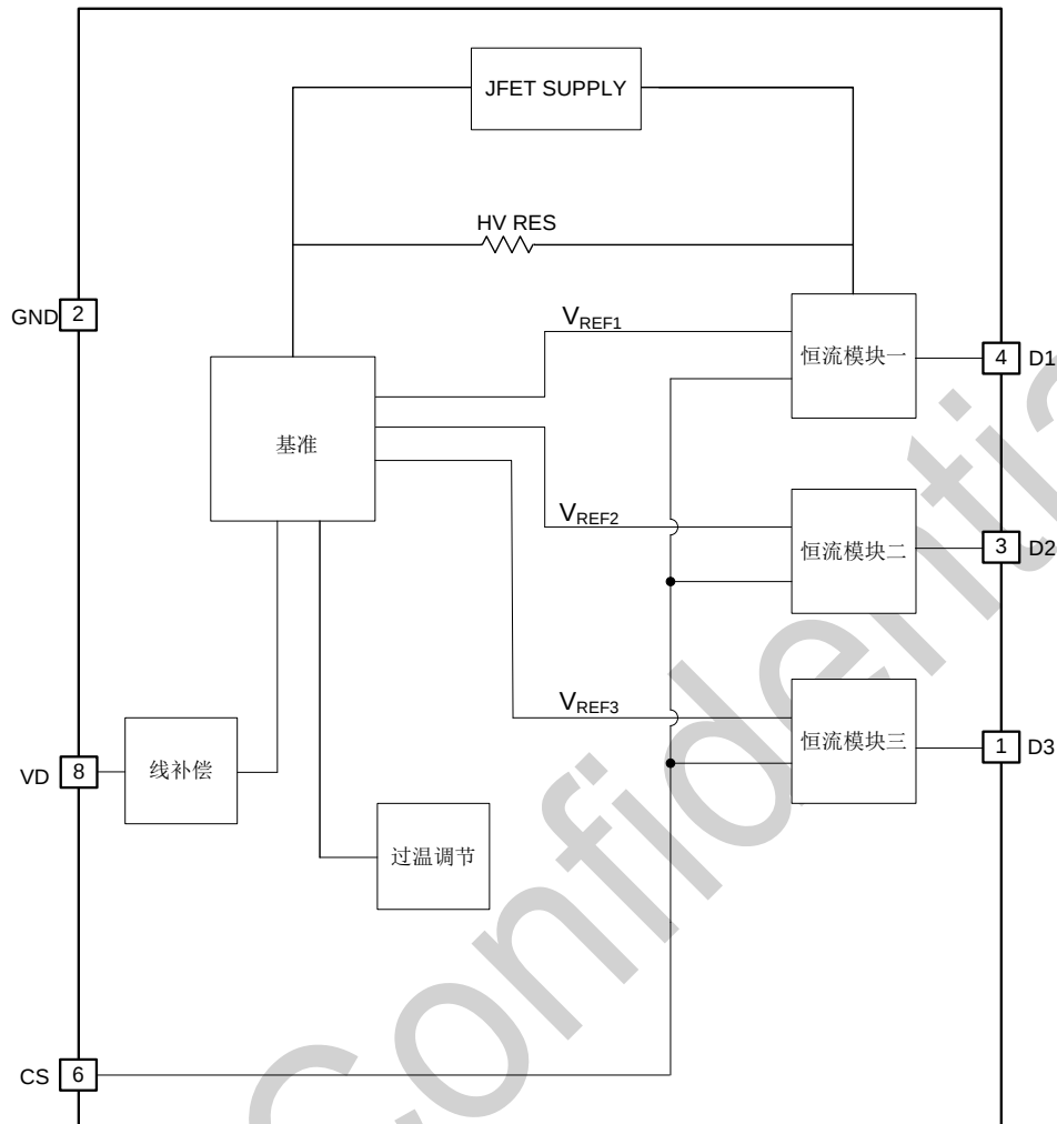
图 3 BP5356HB 内部框图
