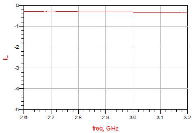
Figure 11. MHC29X03 IL
