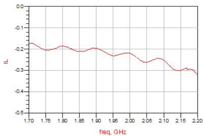
Figure 11. MHC21X02 IL
