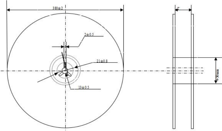
*编带包装盘 (mm)
