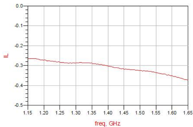
Figure 11. MHC1400C03 IL
