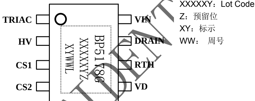
图 2 管脚封装图
