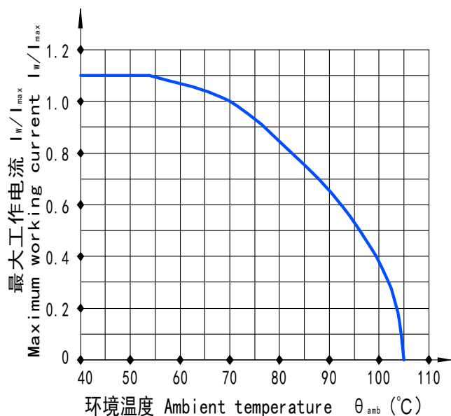
最大工作电流与环境温度关系曲线图
