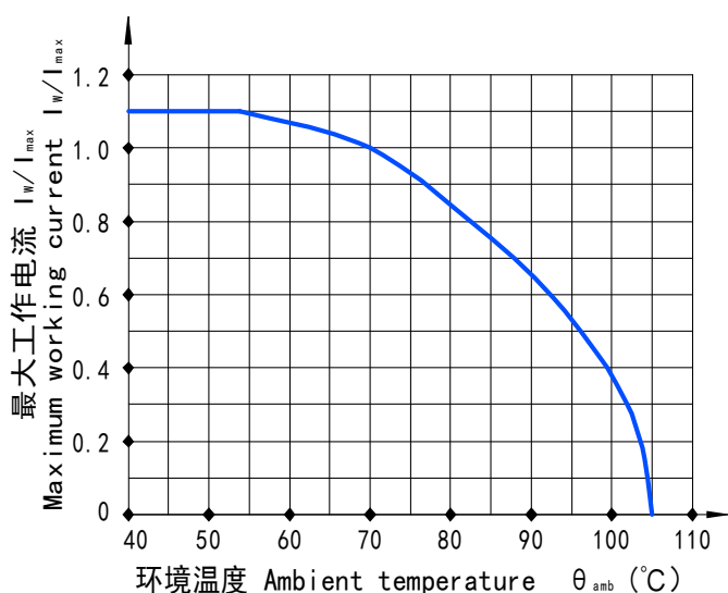
最大工作电流与环境温度关系曲线图
