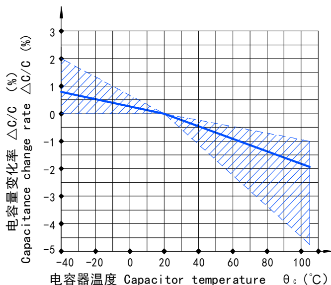
电容量变化率与温度关系曲线图
