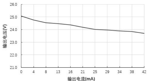
输出电压 VS 输出电流 B0524XT-1WR3@Vin=5V
