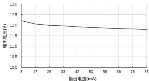
输出电压 VS 输出电流 B2412XT-1WR3@Vin=24V
