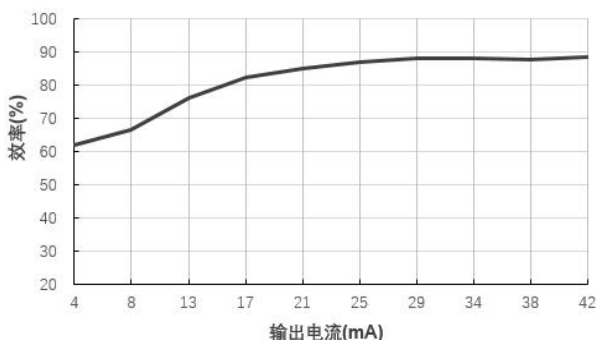
效率 VS 输出电流 B1224XT-1WR3@Vin=12V
