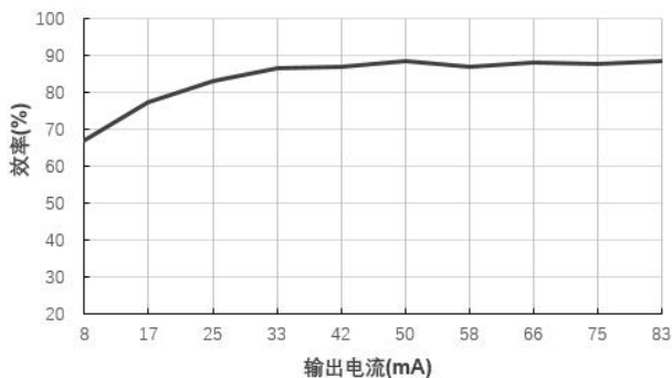
效率 VS 输出电流 B2412XT-1WR3@Vin=24V
