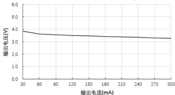
输出电压 VS 输出电流 B0303XT-1WR3@Vin=3.3V
