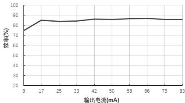
效率 VS 输出电流 B0512XT-1WR3@Vin=5V
