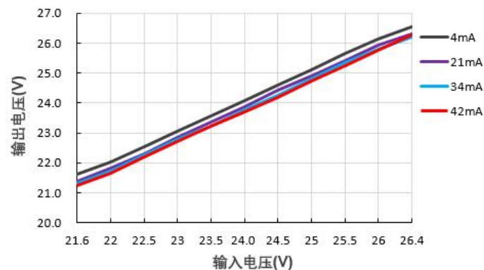
输出电压 VS 输入电压 B2424XT-1WR3@Vin=24V
