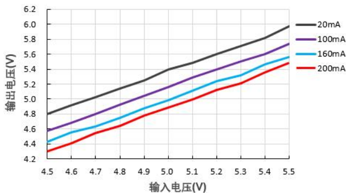
输出电压 VS 输入电压 B0505XT-1WR3@Vin=5V
