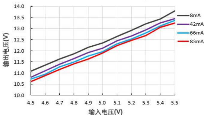
输出电压 VS 输入电压 B0512XT-1WR3@Vin=5V
