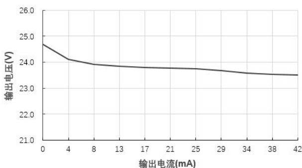
输出电压 VS 输出电流 B1224XT-1WR3@Vin=12V
