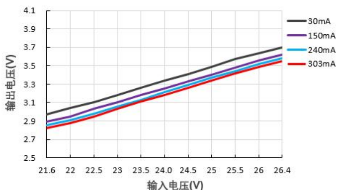
输出电压 VS 输入电压 B2403XT-1WR3@Vin=24V
