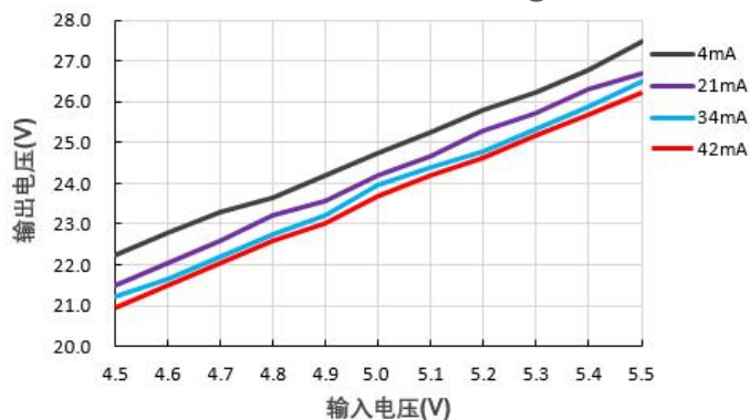
输出电压 VS 输入电压 B0524XT-1WR3@Vin=5V
