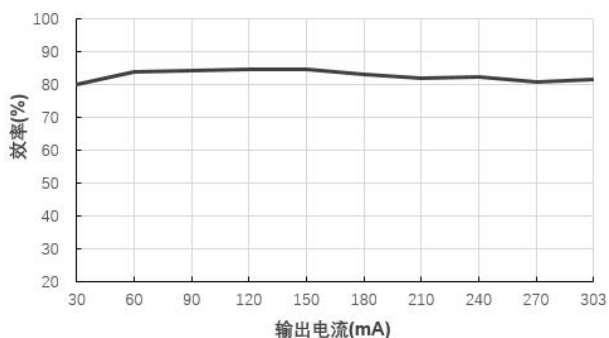
效率 VS 输出电流 B0303XT-1WR3@Vin=3.3V
