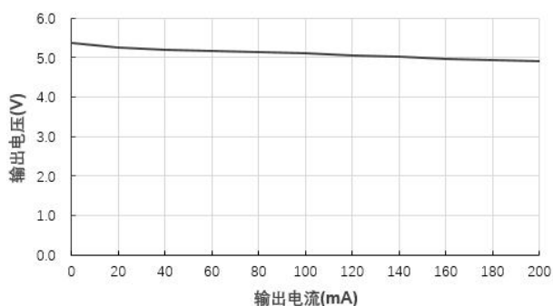
输出电压 VS 输出电流 B1205XT-1WR3@Vin=12V
