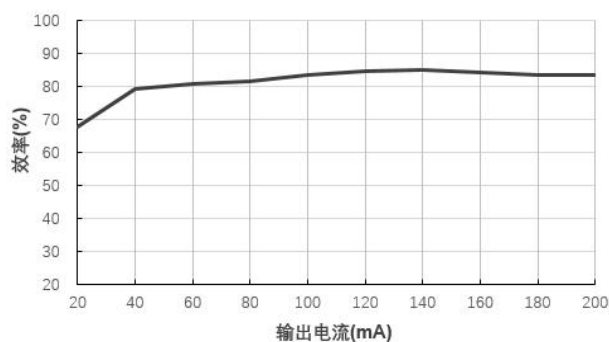
效率 VS 输出电流 B1205XT-1WR3@Vin=12V
