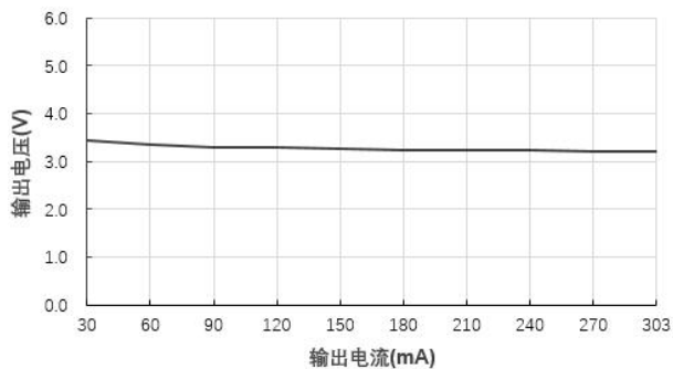
输出电压 VS 输出电流 B2403XT-1WR3@Vin=24V
