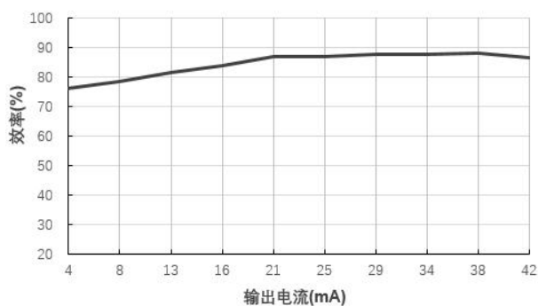
效率 VS 输出电流 B0524XT-1WR3@Vin=5V
