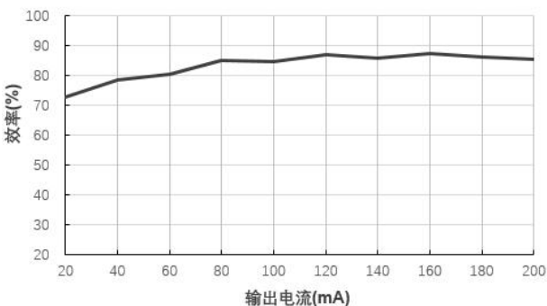
效率 VS 输出电流 B2405XT-1WR3@Vin=24V
