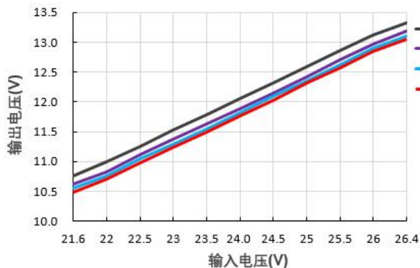
输出电压 VS 输入电压 B2412XT-1WR3@Vin=24V
