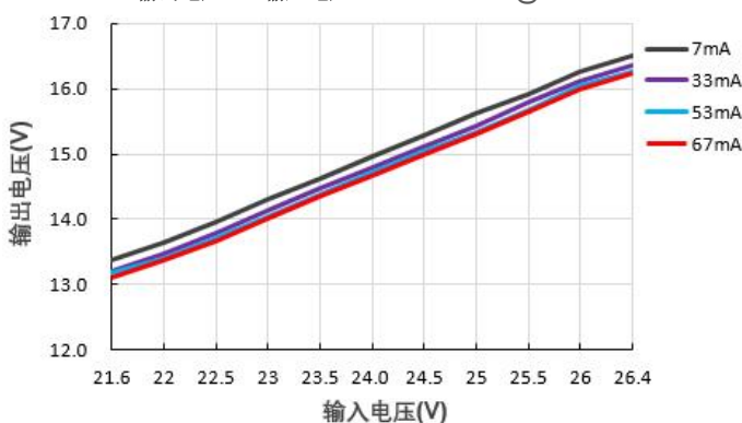
输出电压 VS 输入电压 B2415XT-1WR3@Vin=24V
