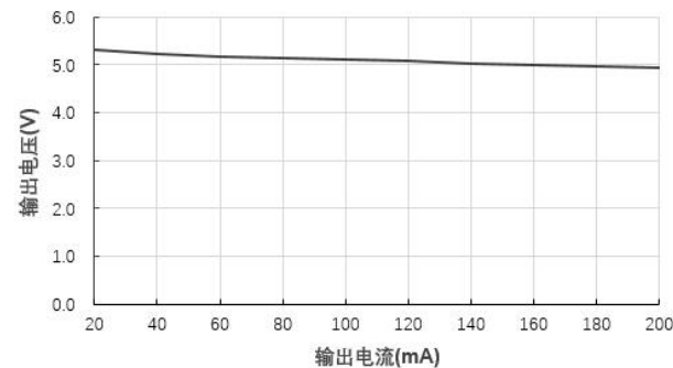
输出电压 VS 输出电流 B2405XT-1WR3@Vin=24V
