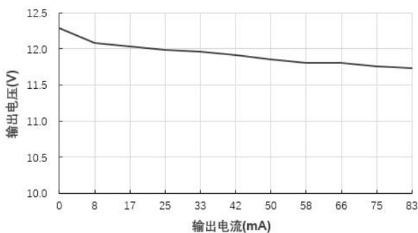
输出电压 VS 输出电流 B1212XT-1WR3@Vin=12V
