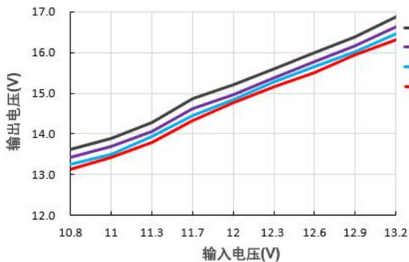
输出电压 VS 输入电压 B1215XT-1WR3@Vin=12V
