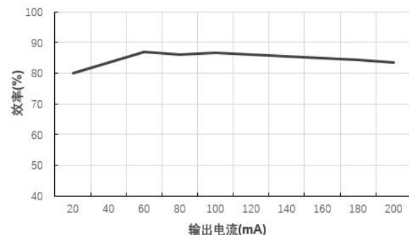
效率 VS 输出电流 B0505XT-1WR3@Vin=5V
