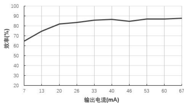
效率 VS 输出电流 B0515XT-1WR3@Vin=5V
