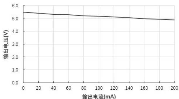
输出电压 VS 输出电流 B0505XT-1WR3@Vin=5V
