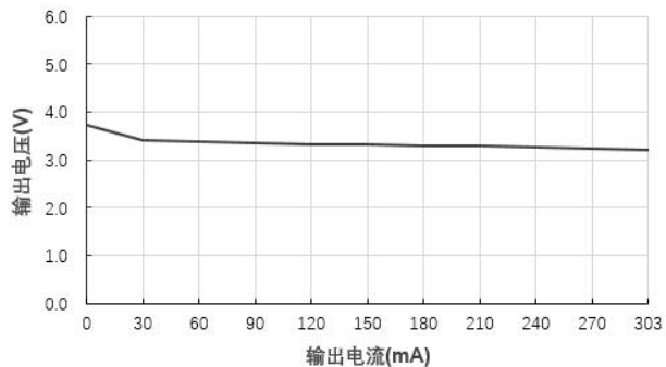
输出电压 VS 输出电流 B1203XT-1WR3@Vin=12V
