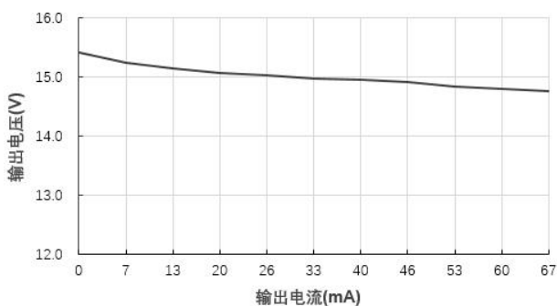
输出电压 VS 输出电流 B1215XT-1WR3@Vin=12V
