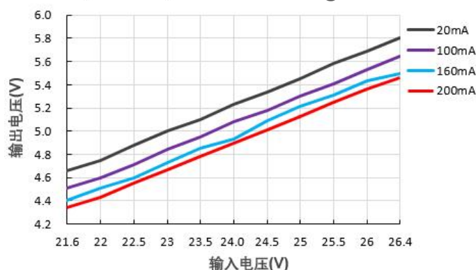
输出电压 VS 输入电压 B2405XT-1WR3@Vin=24V
