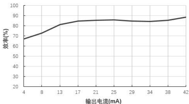
效率 VS 输出电流 B2424XT-1WR3@Vin=24V
