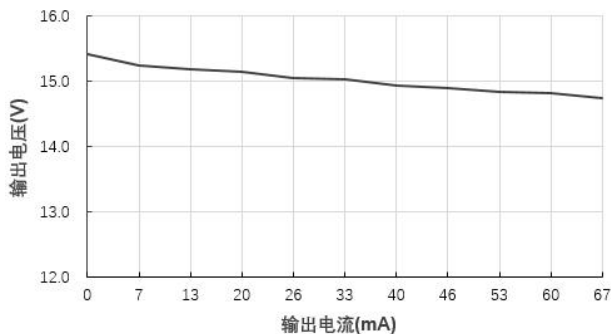
输出电压 VS 输出电流 B0515XT-1WR3@Vin=5V
