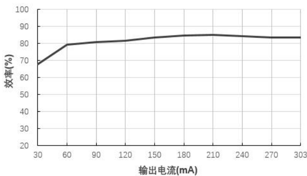
效率 VS 输出电流 B1203XT-1WR3@Vin=12V
