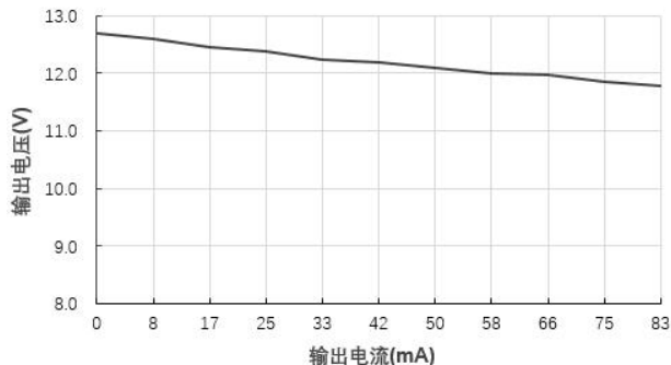
输出电压 VS 输出电流 B0512XT-1WR3@Vin=5V
