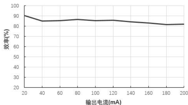
效率 VS 输出电流 B0305XT-1WR3@Vin=3.3V
