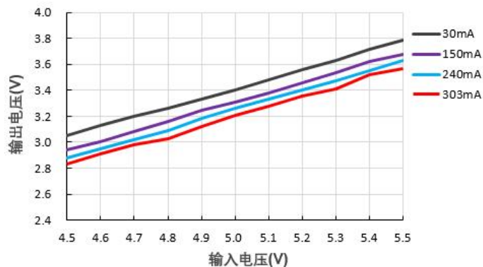
输出电压 VS 输入电压 B0503XT-1WR3@Vin=5V
