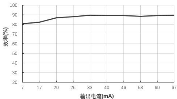
效率 VS 输出电流 B1215XT-1WR3@Vin=12V
