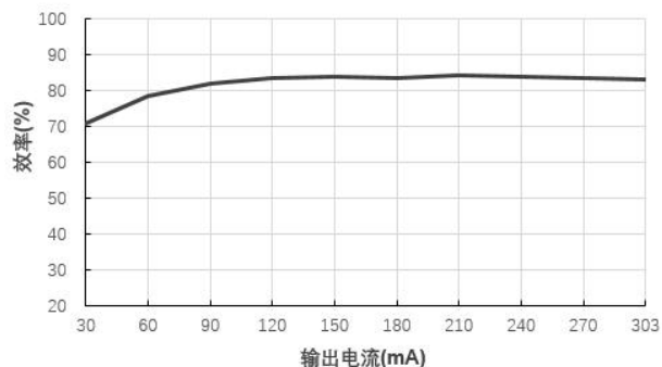
效率 VS 输出电流 B0503XT-1WR3@Vin=5V
