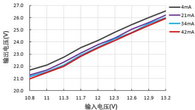
输出电压 VS 输入电压 B1224XT-1WR3@Vin=12V
