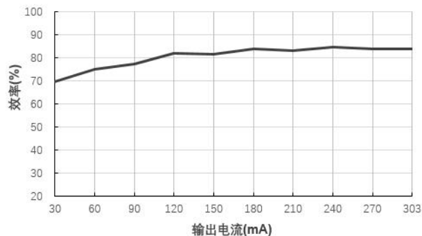
效率 VS 输出电流 B2403XT-1WR3@Vin=24V
