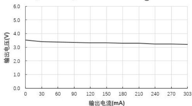
输出电压 VS 输出电流 B0503XT-1WR3@Vin=5V
