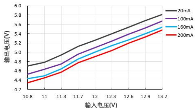
输出电压 VS 输入电压 B1205XT-1WR3@Vin=12V
