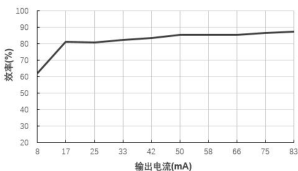
效率 VS 输出电流 B1212XT-1WR3@Vin=12V
