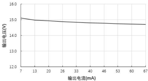
输出电压 VS 输出电流 B2415XT-1WR3@Vin=24V
