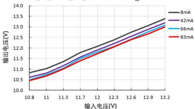
输出电压 VS 输入电压 B1212XT-1WR3@Vin=12V
