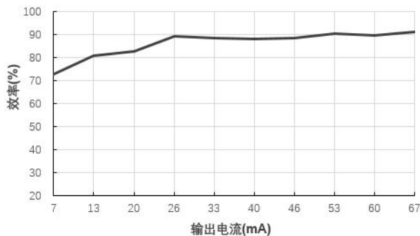
效率 VS 输出电流 B2415XT-1WR3@Vin=24V
