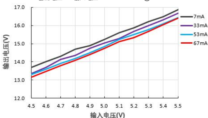
输出电压 VS 输入电压 B0515XT-1WR3@Vin=5V
