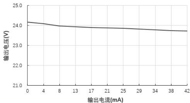
输出电压 VS 输出电流 B2424XT-1WR3@Vin=24V
