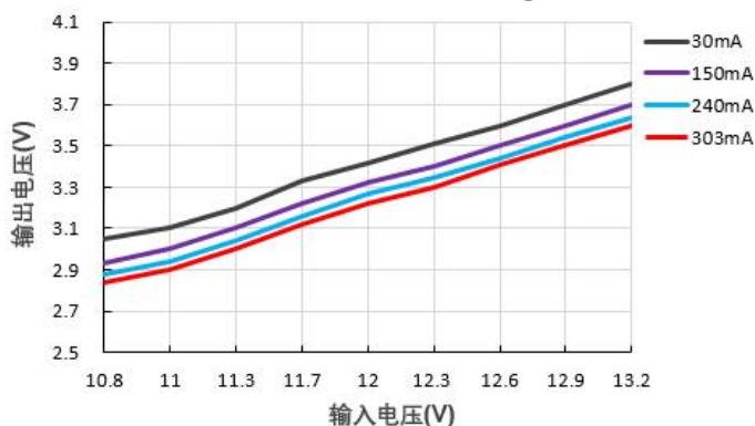
输出电压 VS 输入电压 B1203XT-1WR3@Vin=12V
