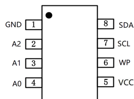
SOT-23-8
