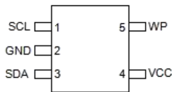
SOT-23-5
