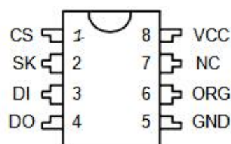
DIP-8
