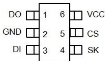
SOT-23-6
