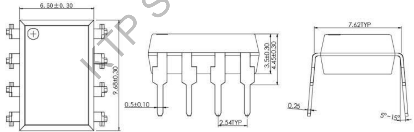
FOD3182-C1H0 DIP8 外形尺寸
