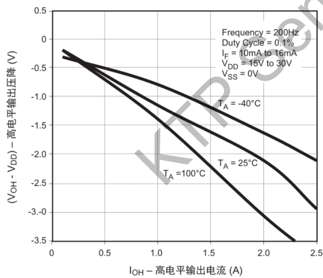
图 1.高电平输出电压降 vs.高电平输出电流
