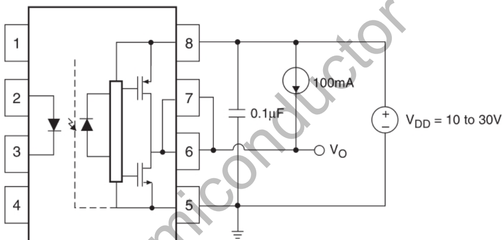
图 23. V_{OL} 测试电路
