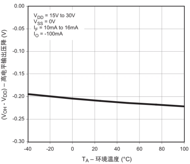
图 2.高电平输出电压降 vs.环境温度
