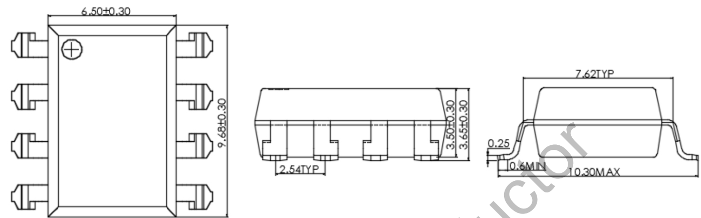
FOD3182-C5H0 SMD8 外形尺寸
