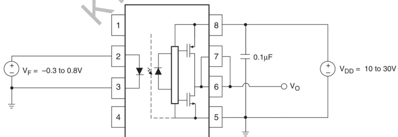
图 27. V_{FHL} 测试电路
