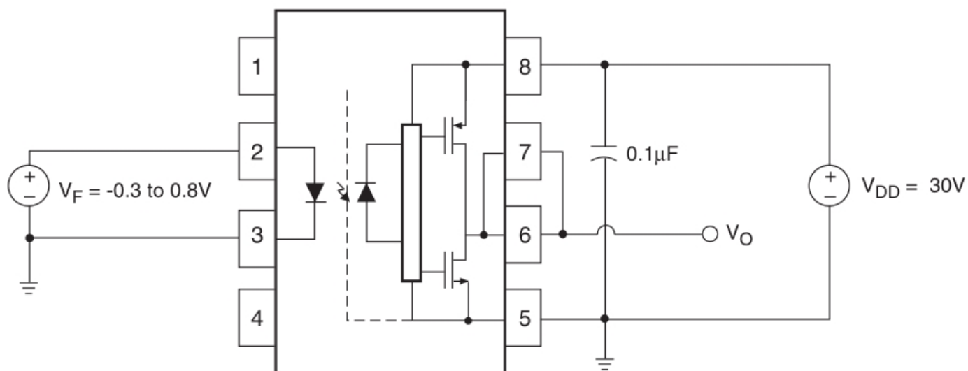
图 25. I_{DDL} 测试电路
