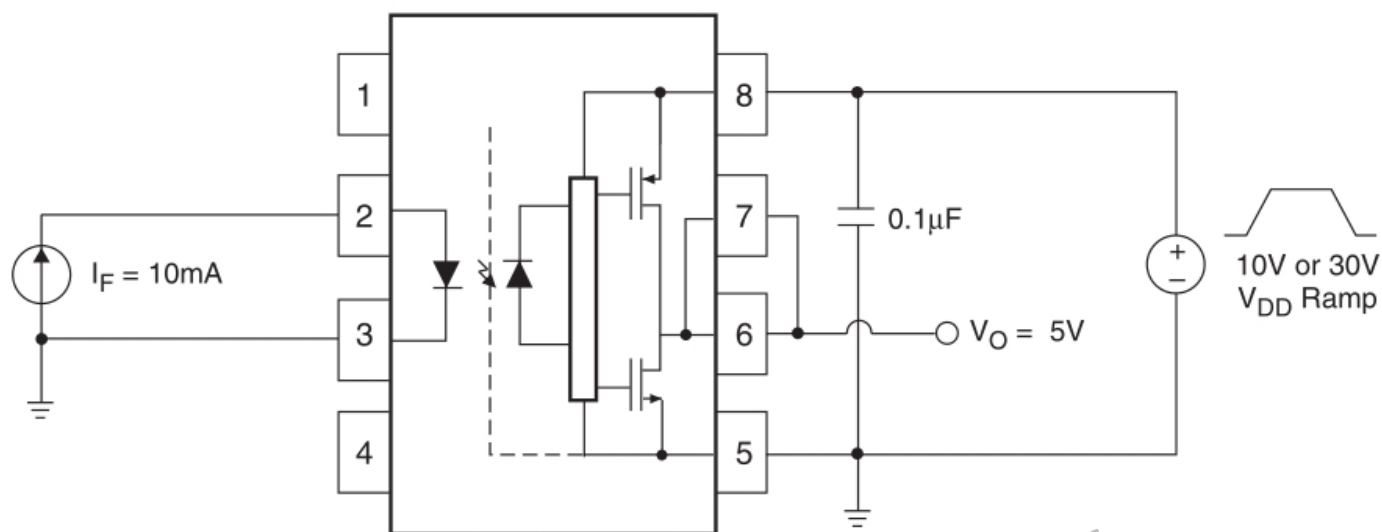
图 28. UVLO 测试电路
