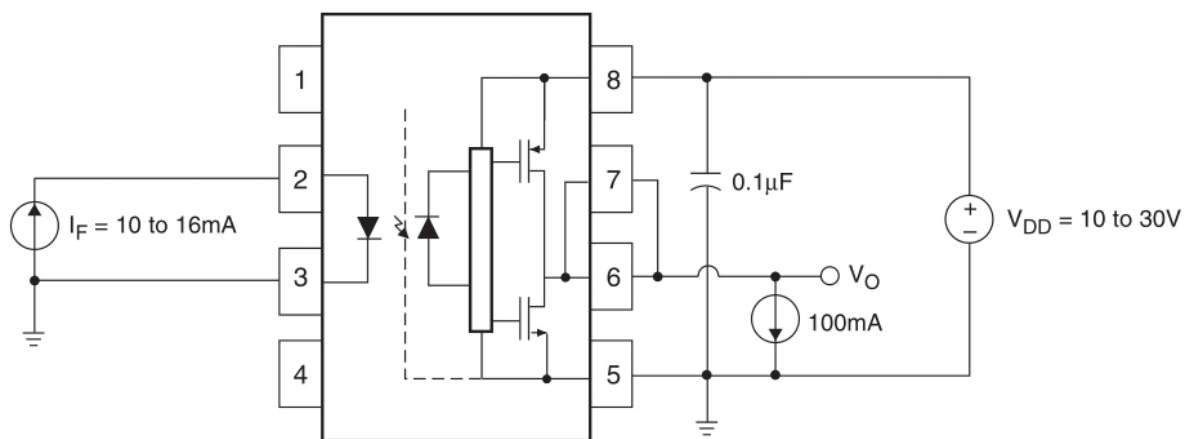
图 22. V_{OH} 测试电路
