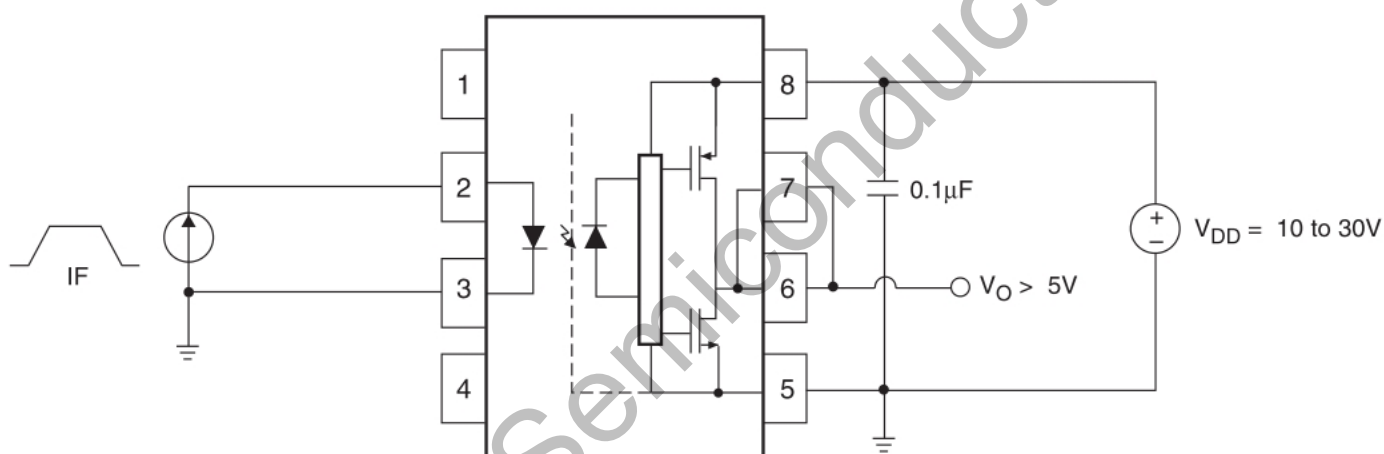
图 26. I_{FLH} 测试电路
