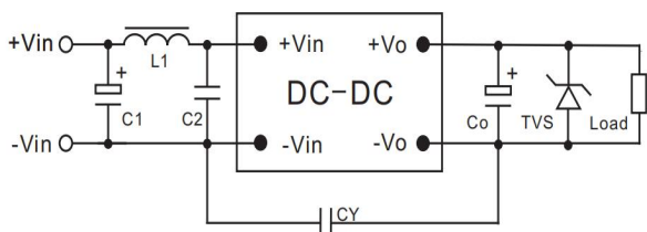
(1) 典型应用电路（一）：
