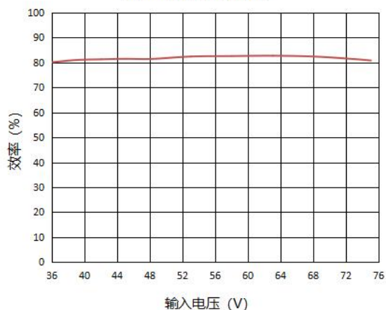
效率VS输入电压 (满载)
