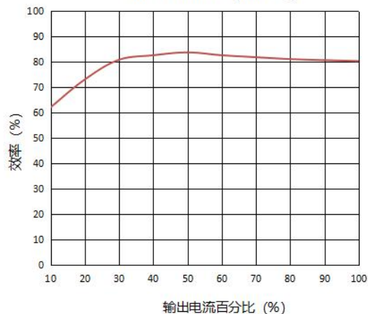
效率VS输出负载 (48V输入)
