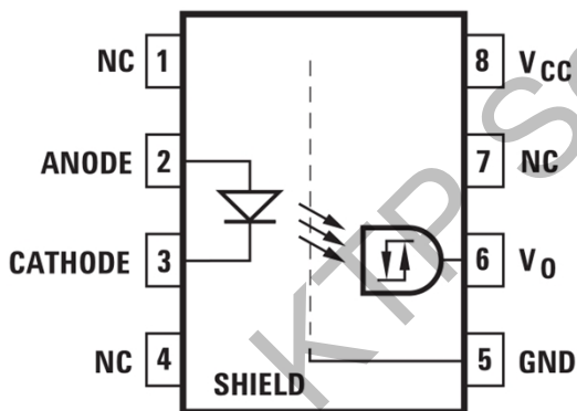
ACPL-4800 功能框图 (2)
