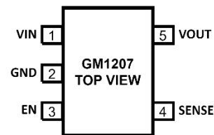
图 4.8 引脚 SOT-23 的引脚配置
