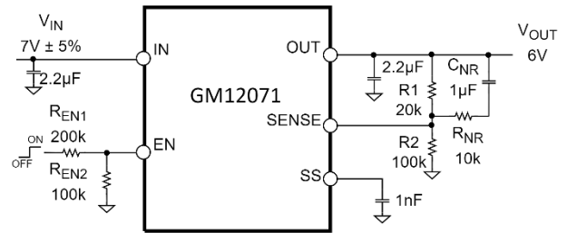
图 30. 噪声优化
