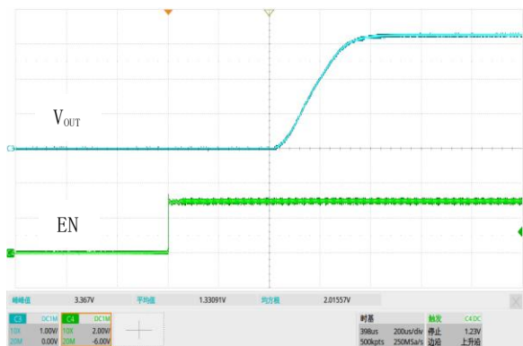
图 23. 软启动, V_{IN}=4.3V , V_{OUT}=3.3V , I_{OUT}=500mA
