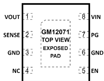
图 5.8 引脚 DFN 的引脚配置
