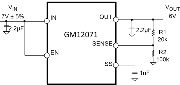
图 26. 典型可调输出电压应用原理图
