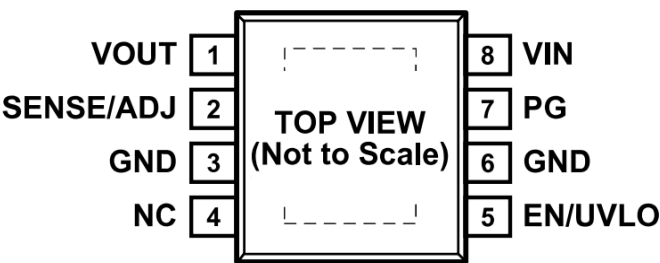
图 6.8 引脚 SOP-8 的引脚配置
