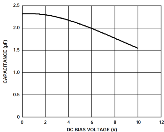
图 27. 电容与电压关系特性
