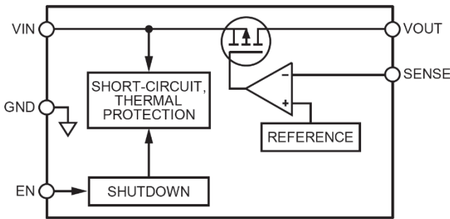
图 25. 内部框图
