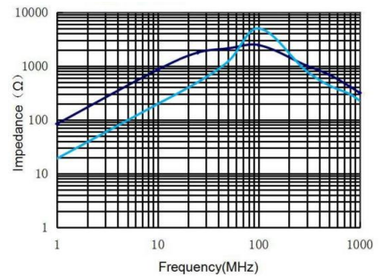
CMF9070F-701-2P-T
