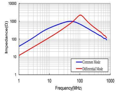
CMF1513F-701-2P-T
