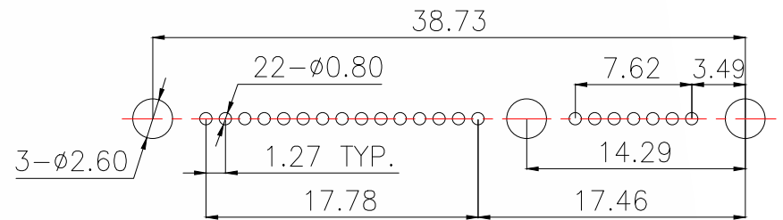
P.C.B LAYOUT
