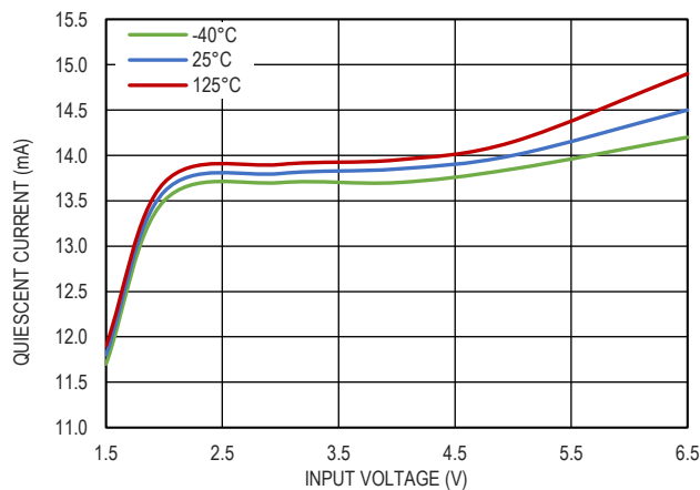
图 7. 静态电流和输入电压的关系, I_{OUT}=1mA
