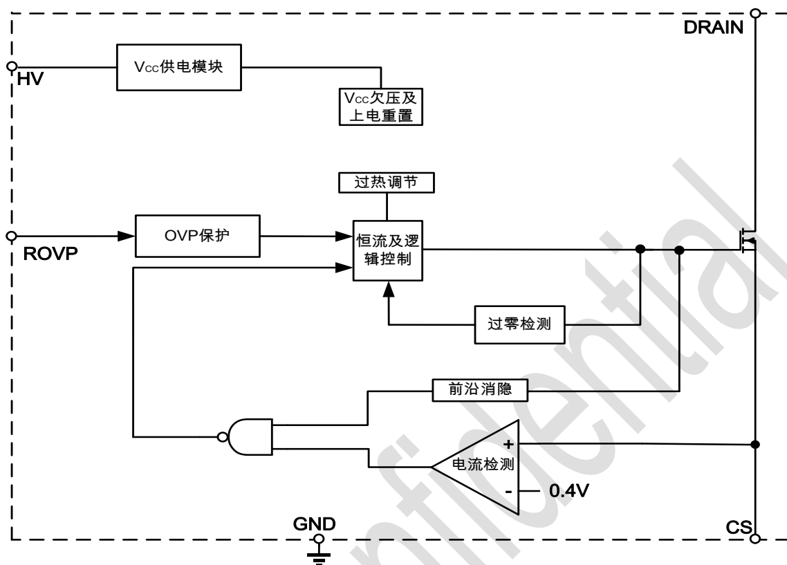
图 3 BP3167XH 系列内部框图
