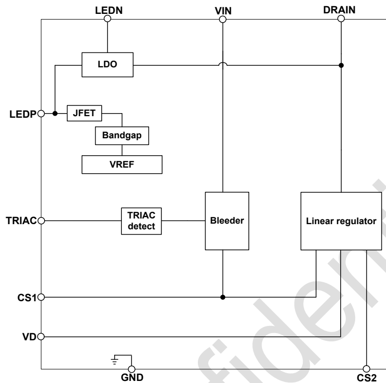
图 3 BP5178BCX 内部框图
